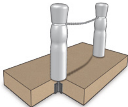
Einfundamentierung des Begrenzungspfostens mit Hilfe des Bodenankers auf losem Untergrund.
