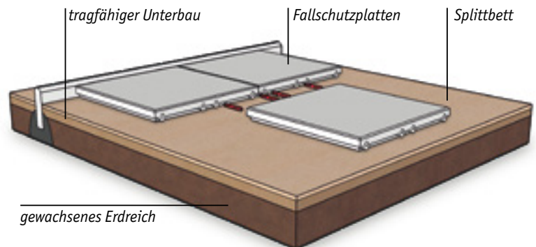
Verlegung auf sickerfähigen Untergründen und im Halbverband mit den Systemsteckern
