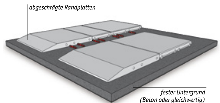
Verlegung auf festen Untergründen und im Halbverband mit Hilfe der Systemstecker
